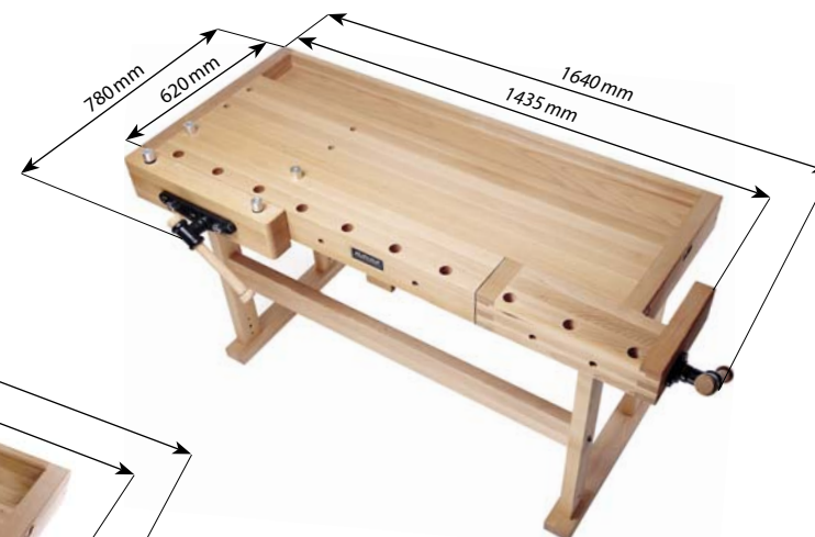
SHORT version of PREMIUM PLUS workbench KURZE Version der PREMIUM PLUS Werkbank
