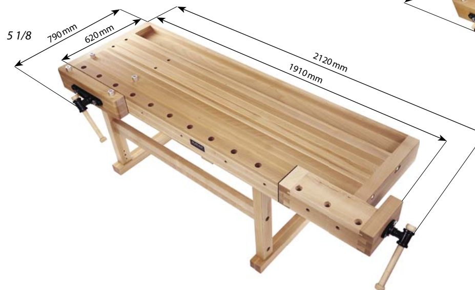
SHORT version of PREMIUM MONSTER workbench KURZE Version der PREMIUM MONSTER Werkbank
