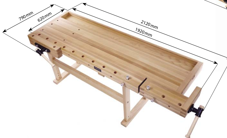
LONG version of PREMIUM PLUS workbench LANGE Version der PREMIUM PLUS Werkbank
