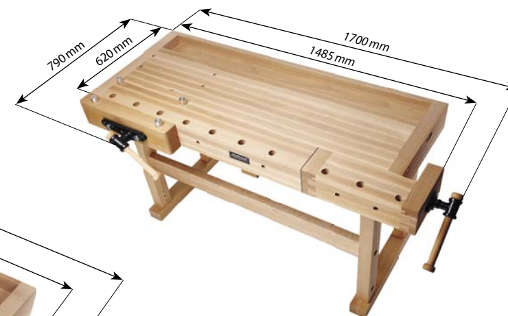
SHORT version of PREMIUM MONSTER workbench KURZE Version der PREMIUM MONSTER Werkbank
