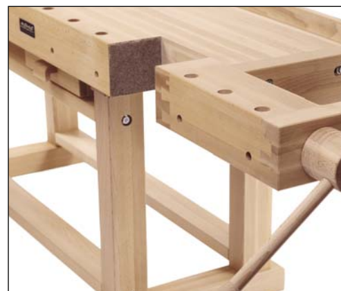
Opening capacity 145 mm / 5 45 / 64 in Öffnungskapazität 145 mm
