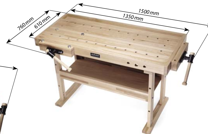
SHORT version of DIAMOND workbench KURZE Version der DIAMOND Werkbank
